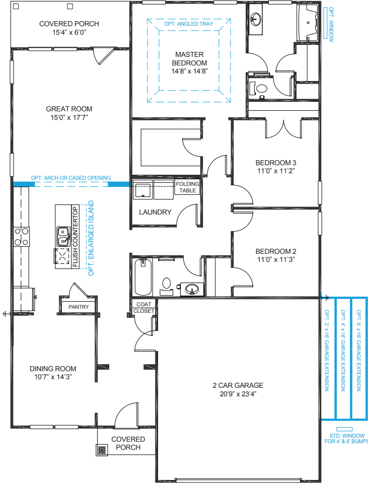
Plan 1760
