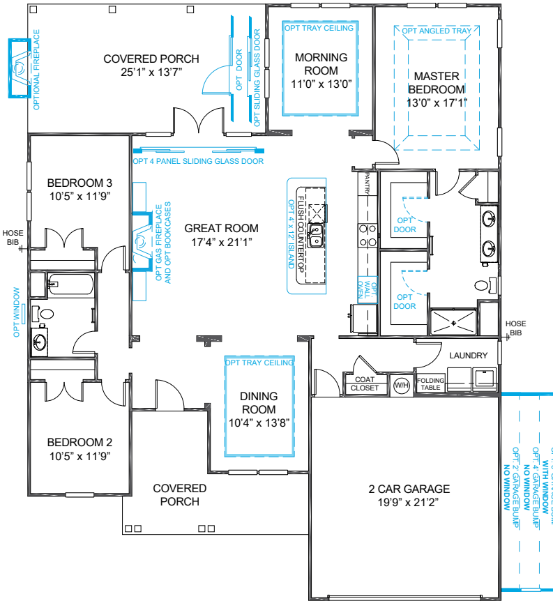
Plan 2112
